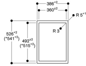
Yukarıdan görünüm
