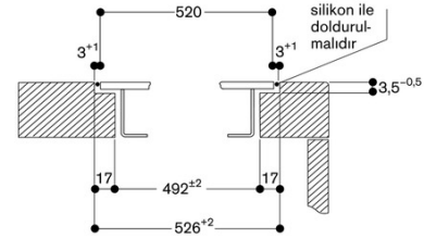
Çapraz kesit
