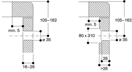
Kumanda düğmesi montajı, yüzeye montaj
