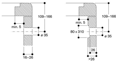
Kumanda düğmesi montajı, yüzeye silme montaj
