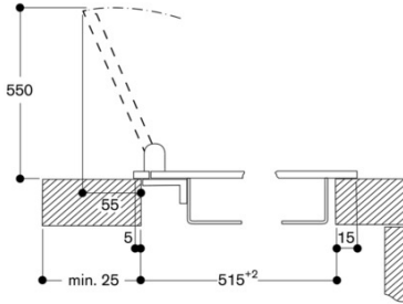
Cihaz kapağı / dengeleme çitası ile montaj, üst üste montaj
