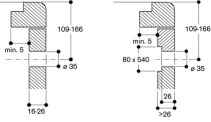
Kumanda düğmesi montajı, yüzeye silme montajı
